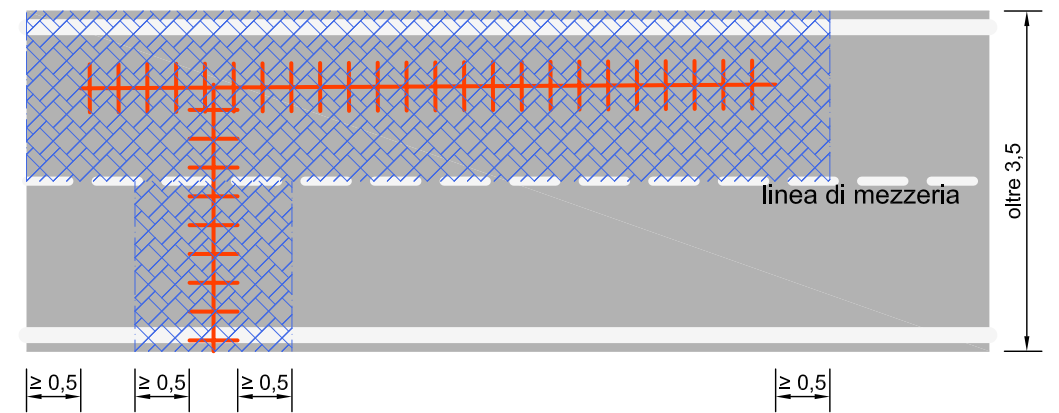
FIGURA 12 - scavi multipli
