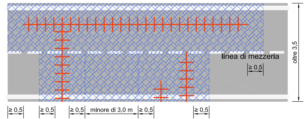
FIGURA 13 - scavi multipli
