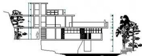
CORTE B - B
