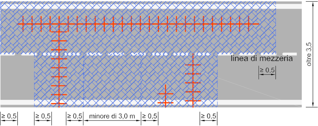
FIGURA 13 - scavi multipli
