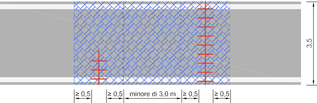
FIGURA 5 - scavi multipli
