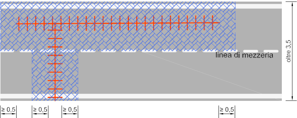
FIGURA 12 - scavi multipli
