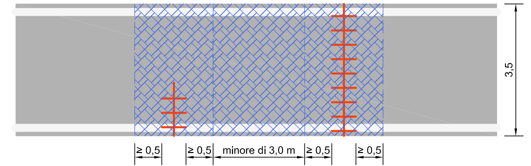
FIGURA 5 - scavi multipli
